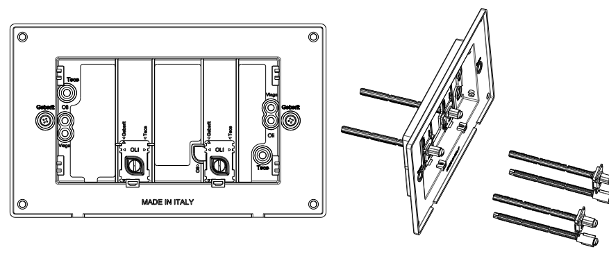
KIT103-Viega: 2H-2L-1F-1C
