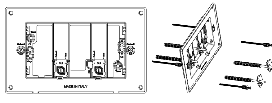
KIT103-Viega: 2H-2L-1F-1C
