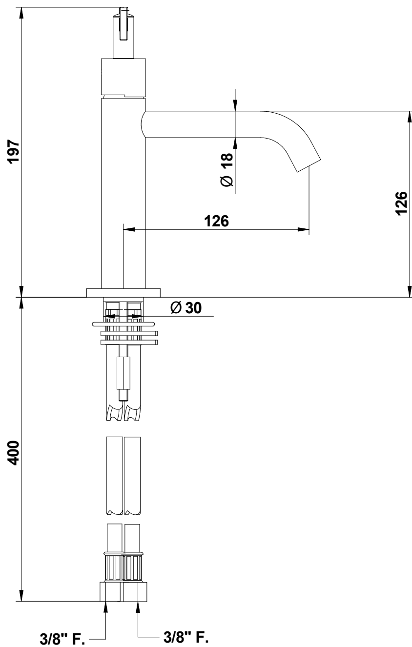
Miscelatore lavabo con cartuccia tradizionale
