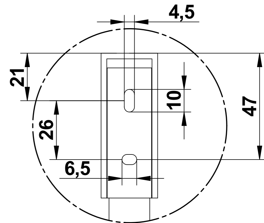
DETTAGLIO A
