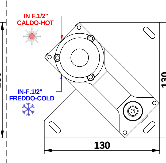
POSIZIONE INCASSO - C BUILT-IN POSITION
