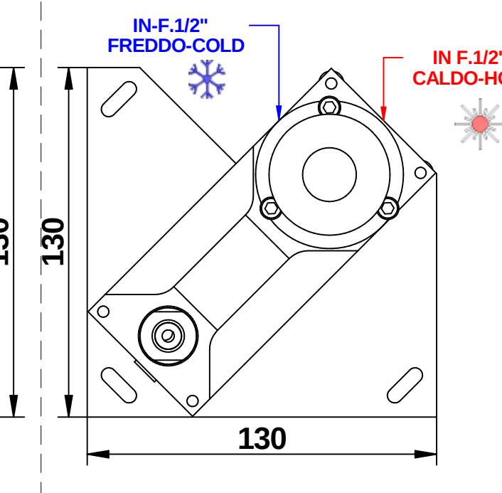
POSIZIONE INCASSO - D BUILT-IN POSITION
