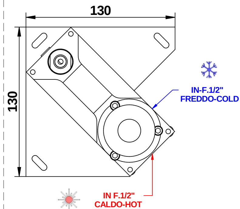
POSIZIONE INCASSO - A BUILT-IN POSITION
