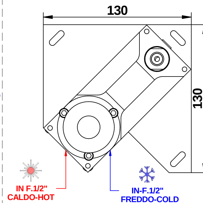
POSIZIONE INCASSO - B BUILT-IN POSITION
