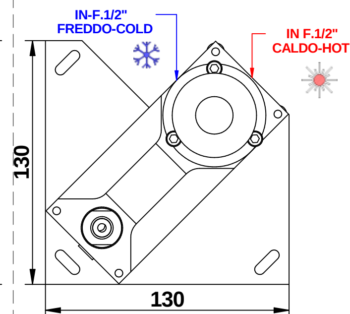
POSIZIONE INCASSO - D BUILT-IN POSITION
