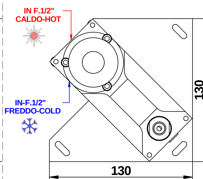
POSIZIONE INCASSO - C BUILT-IN POSITION
