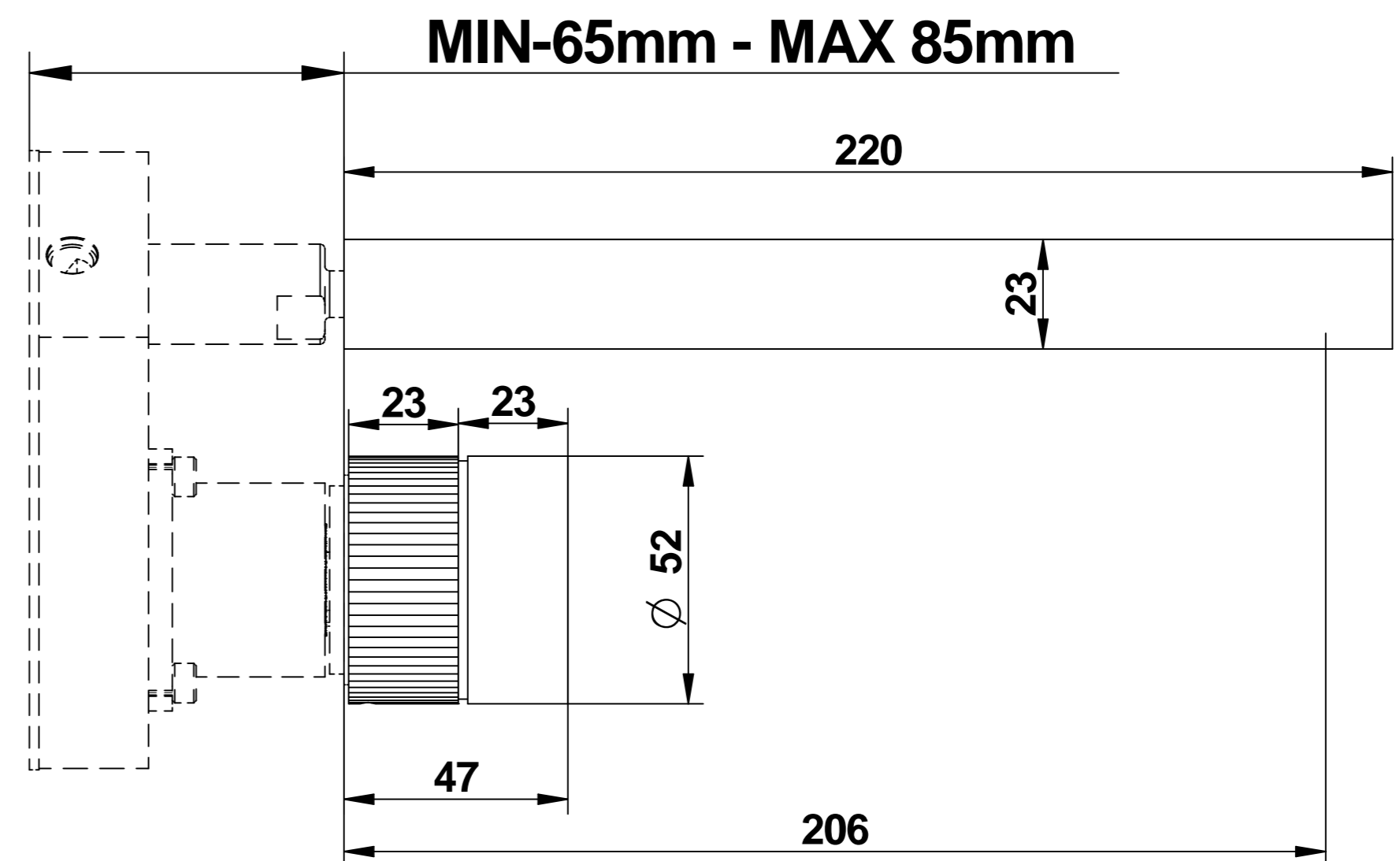
POSIZIONE INCASSO - B BUILT-IN POSITION
