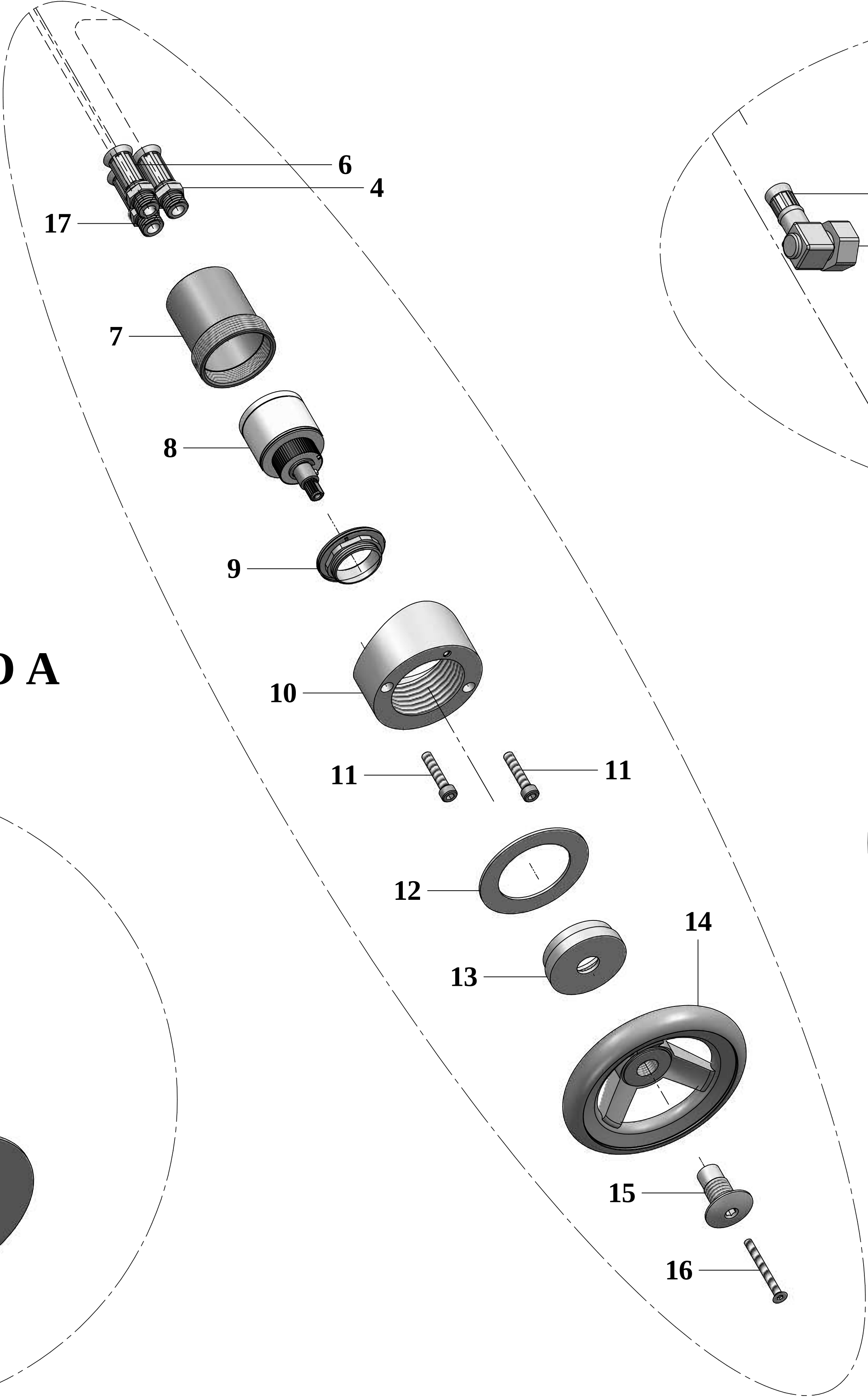
DETTAGLIO B
