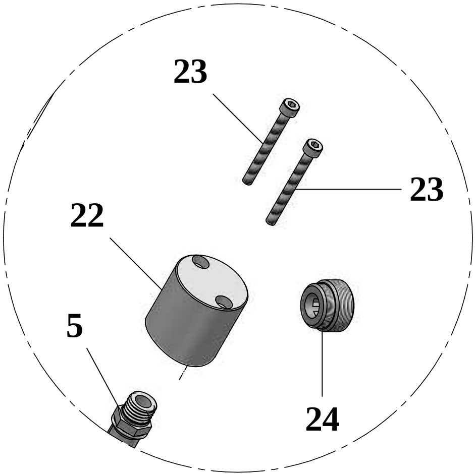
DETTAGLIO E
