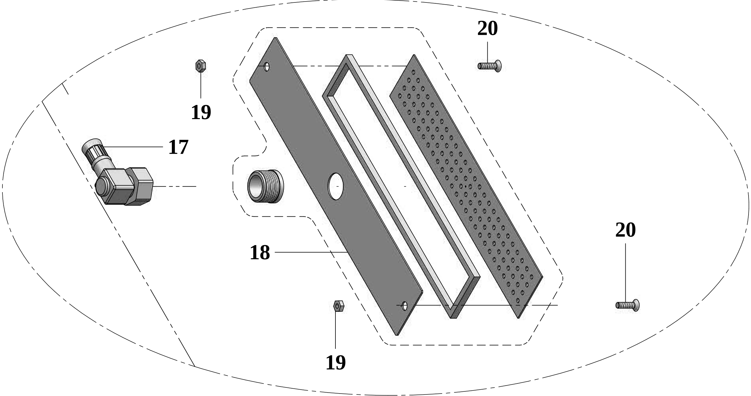
DETTAGLIO C
