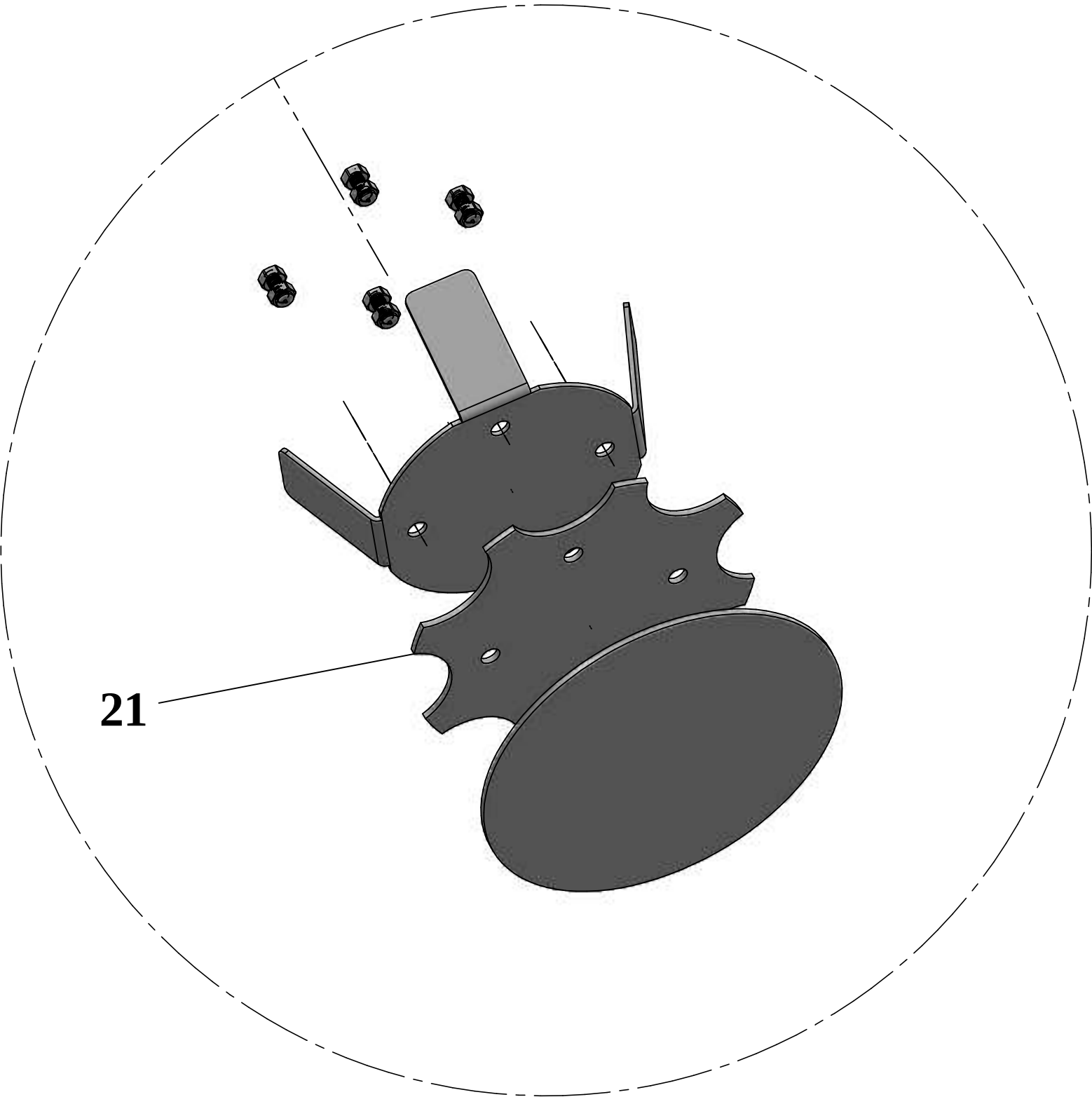
DETTAGLIO D
