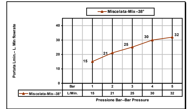
PORTATE A PRESSIONE DINAMICA SENZA LIMITATORE FLOW RATES AT DYNAMIC PRESSURE WITHOUT LIMITATION SYSTEM
